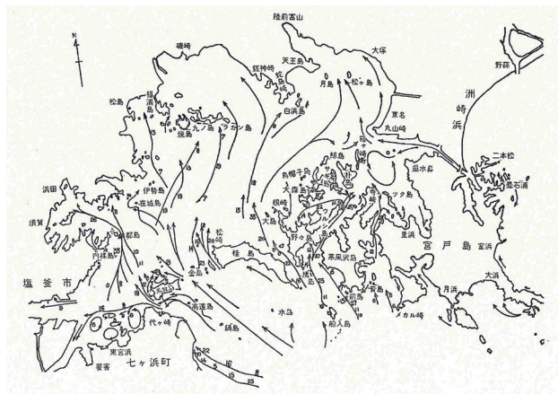
上げ潮時の流跡線 (流速単位: cm/秒)
